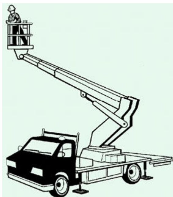
Figura 1 Partes de una plataforma elevadora móvil de personal
