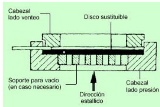
Figura 4. Disco de ruptura plano
