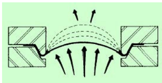
Fig. 1: Disco de ruptura abovedado convencional
