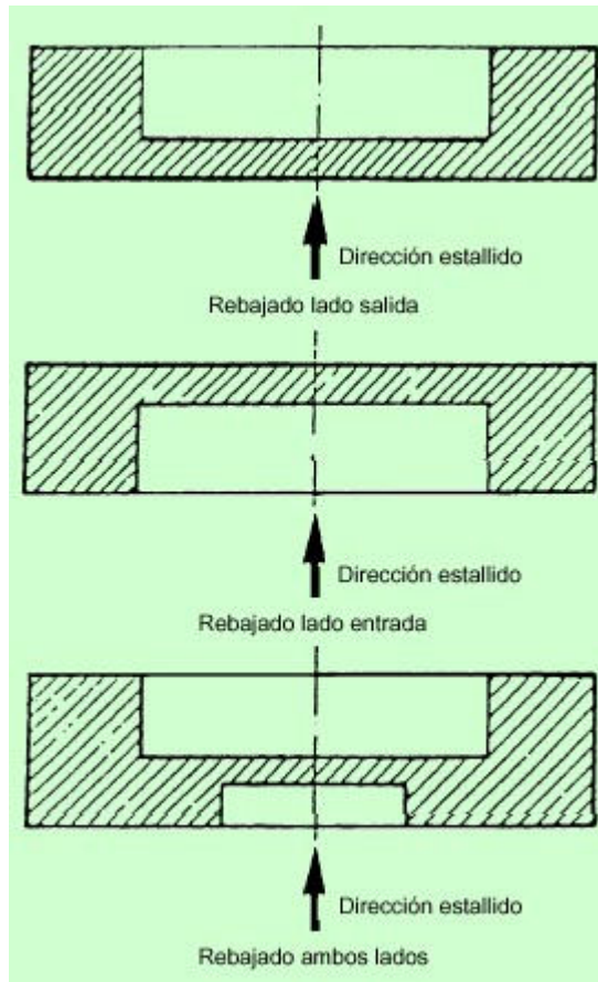
Fig. 5: Disco de ruptura monobloque
