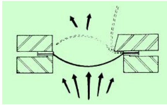
Fig. 2. Disco de ruptura abovedado invertido
