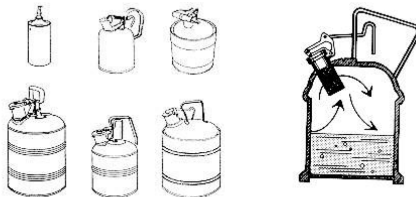
a) Bidones de seguridad provistos de bocas con tapas herméticamente ajustadas o válvulas de mando manual y cierre automático por muelles b) Sección transversal de un recipiente de seguridad dotado de tapa o resorte que descarga la presión interna de vapor a conveniencia
