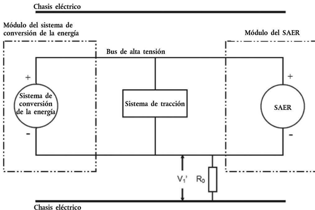
Figura 3 Medición de V_1'
