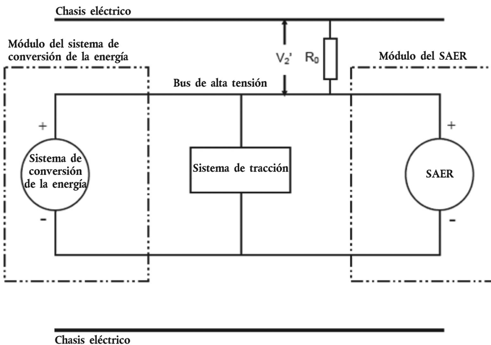
Figura 4 Medición de V_2'
