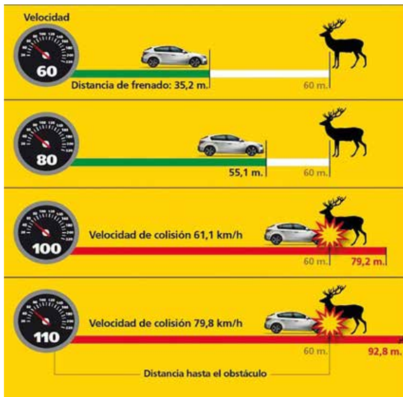
► Distancia de frenado en función de la velocidad
