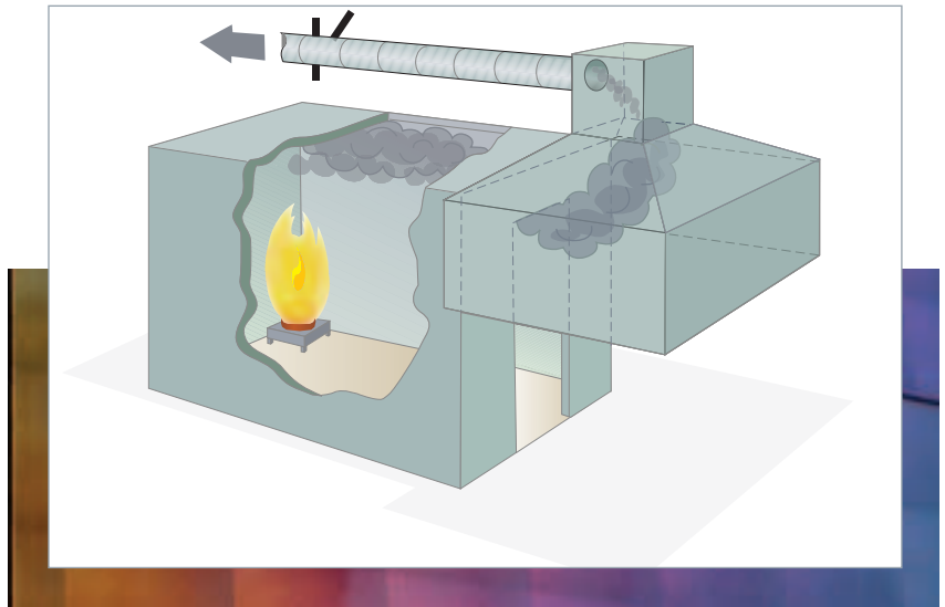
Figura 2. Esquema del ensayo Room/Corner Test (ISO 9705). Fuente: SP –Swedish National Testing & Research Institute.
