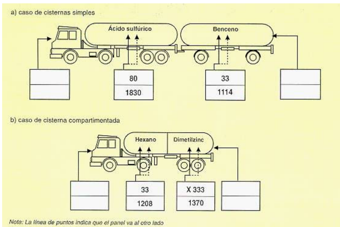
Fig. 1: Modelo de panel según Marginal 250.001
