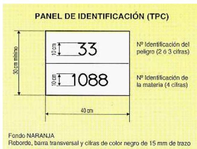
Fig. 1: Modelo de panel según Marginal 250.001
