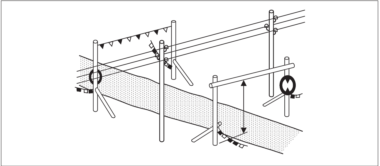
Figura 28 - Ejemplo de sistemas de protección para trabajos en proximidad de líneas aéreas.
