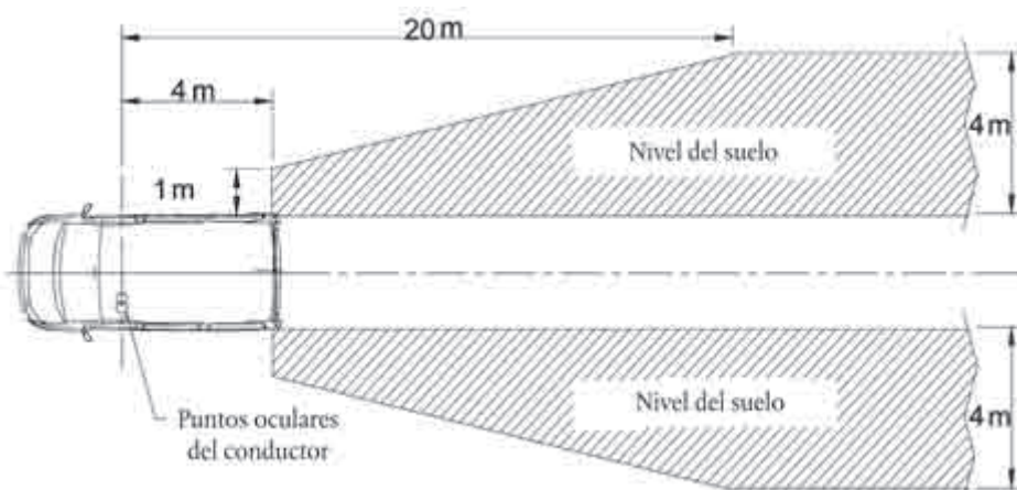
Figura 8: Campo de visión de un retrovisor de la clase III
