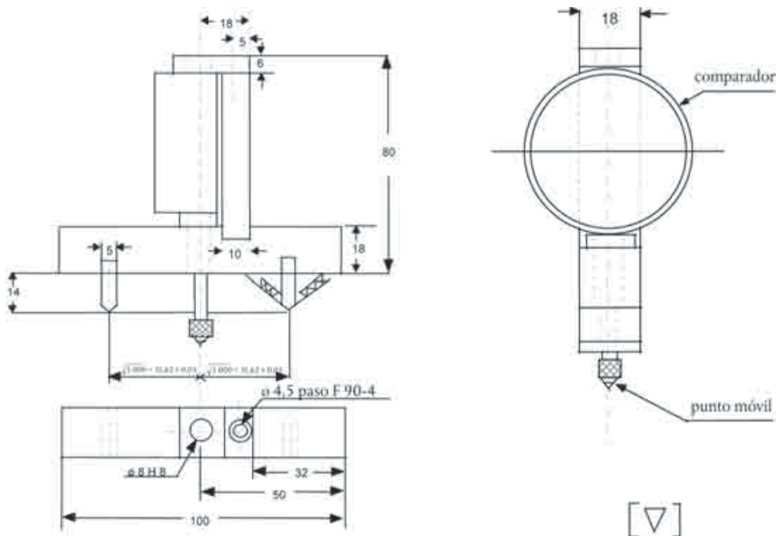
Figura 3: esferómetro
