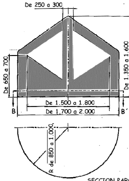
SECCION PARCIAL BB'
