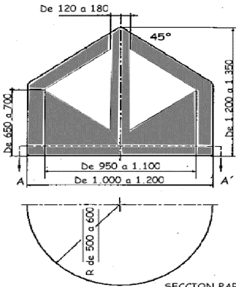
SECCION PARCIAL AA'
