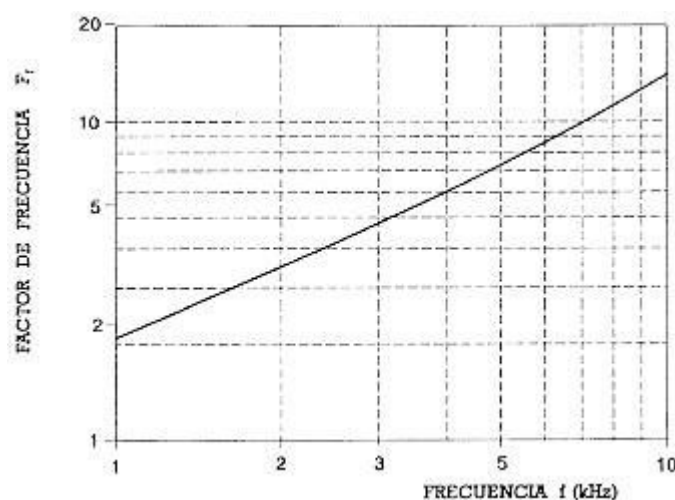
Fig. 6: Umbral de fibrilación. F_f para frecuencias comprendidas entre 1.000 y 10.000 Hz
