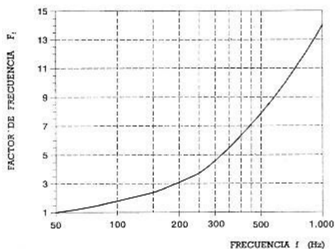
Fig. 5: Umbral de fibrilación. F_f para frecuencias comprendidas entre 50 y 1.000 Hz
