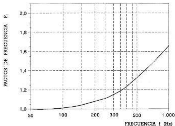
Fig. 4: Umbral de no soltar. F_f para frecuencias comprendidas entre 50 y 1.000 Hz
