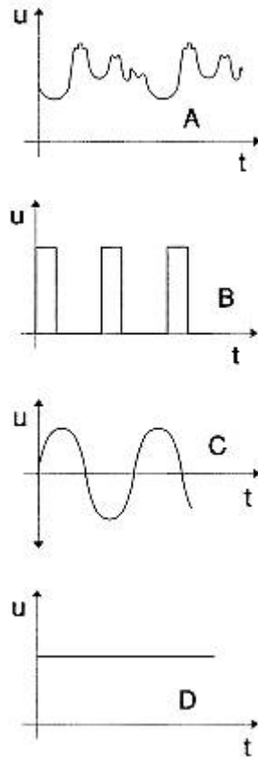
Fig. 1: Ejemplos de forma de onda. A: Señal de televisión, B: Tren de impulsos rectangulares (radar), C: Tensión industrial, D: Tensión constante.
