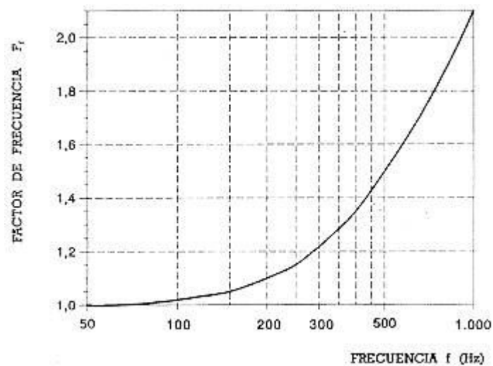
Fig. 3: Umbral de percepción. F_f para frecuencias comprendidas entre 50 y 1.000 Hz
