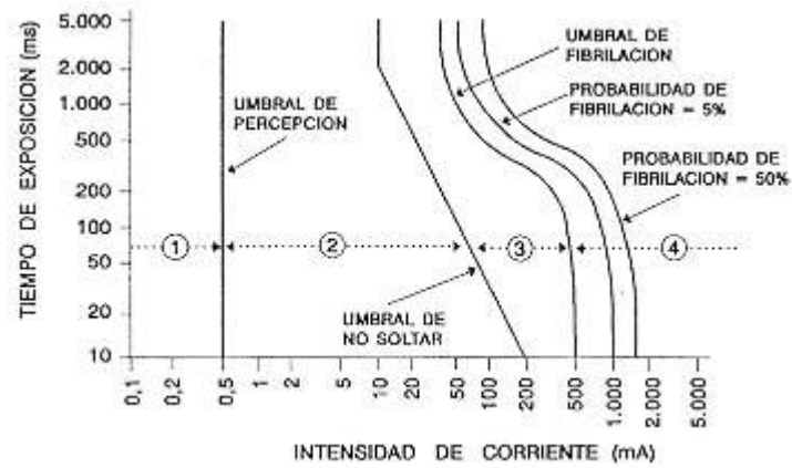
Fig. 2: Efectos de la corriente eléctrica alterna de 50 Hz, en adultos, con trayectoria mano izquierda-los dos pies
