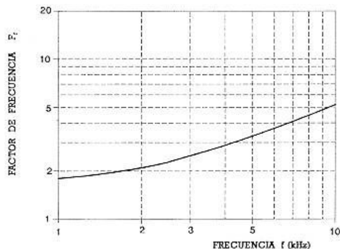
Fig. 7: Umbral de no soltar. F_f para frecuencias comprendidas entre 1.000 y 10.000 Hz
