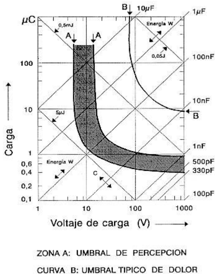
Fig. 12: Umbrales de percepción y de dolor, para una duración de choque de descarga 3T \leq 10 ms, para un trayecto mano-mano, con las manos secas y elevada superficie de contacto
