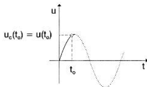
Fig. 9: Estado de carga del condensador al desconectar el circuito
