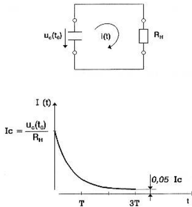
Fig. 10: Descarga de un condensador a través de un individuo de resistencia R_H
