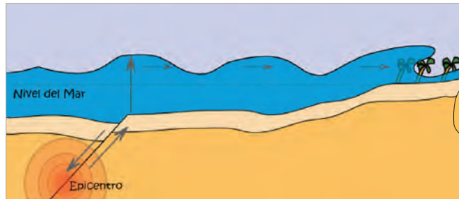
Características físicas de un tsunami
