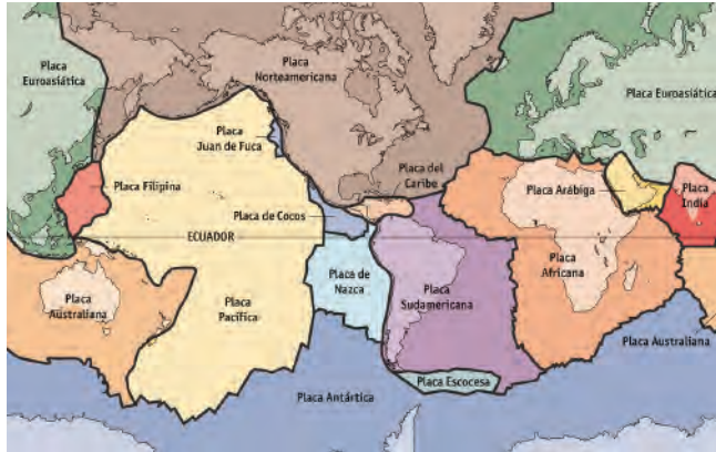
Mapa donde se ven las distintas placas tectónicas
