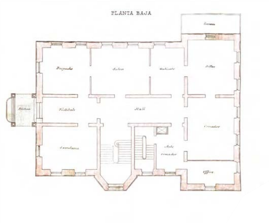
Plano de la planta baja de la casa hotel en la calle Lista nº 16, esquina Lagasca, de Madrid (AVM, expte. casa hotel del marqués de Mochales).
