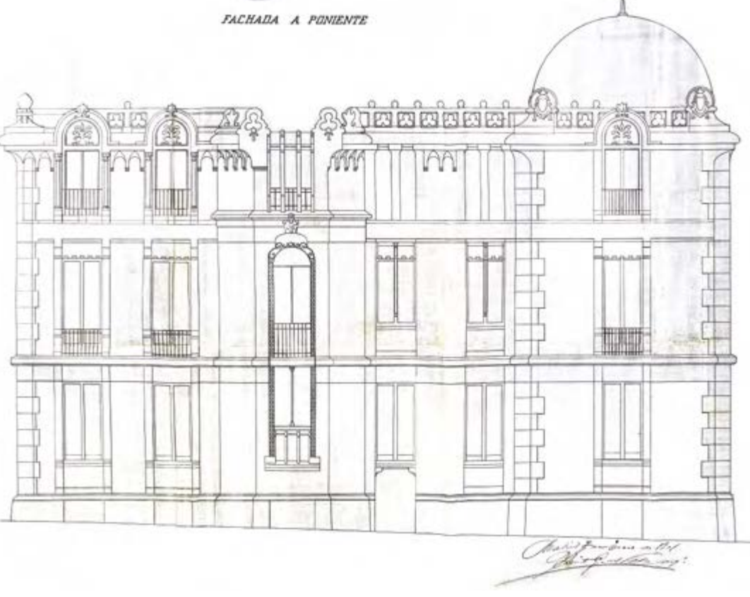
Fachada a poniente de la casa hotel en la calle Lista nº 16, esquina Lagasca, de Madrid.
