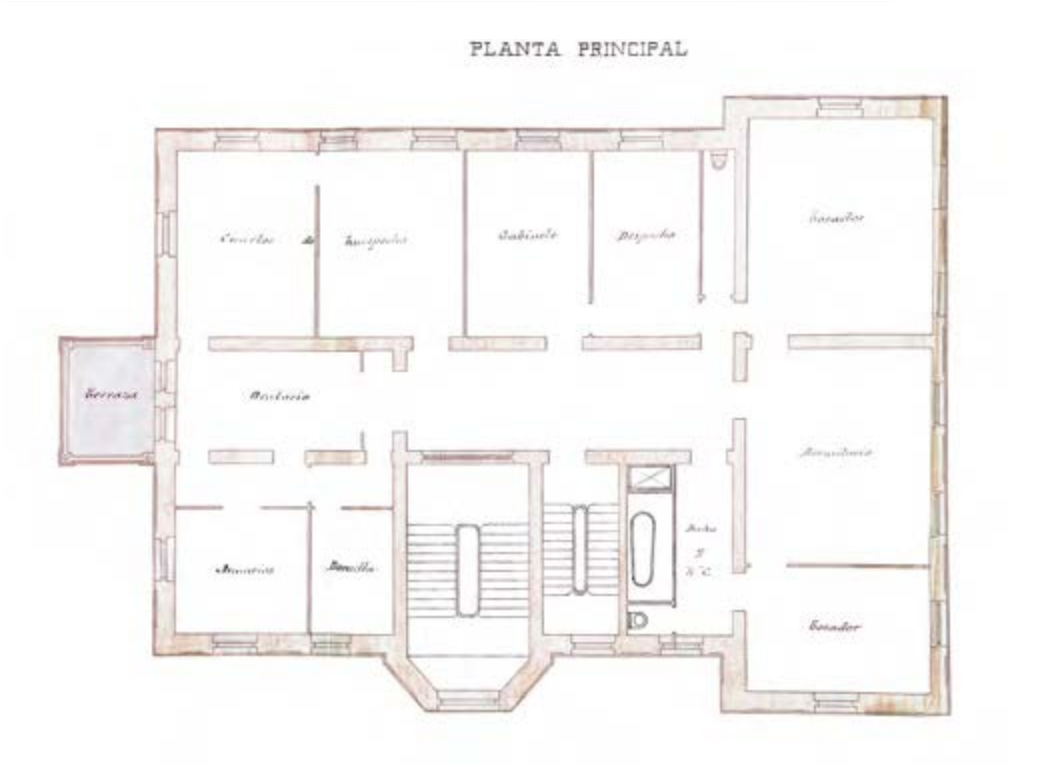
Plano de la planta principal (primer piso) de la casa hotel de los marqueses de Mochales en la calle Lista nº 16 de Madrid, esquina Lagasca (AVM, expte. casa hotel del marqués de Mochales).
