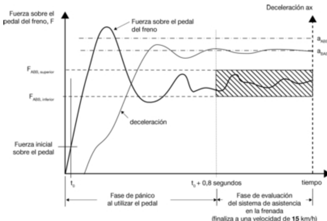
Ejemplo de ensayo 2 de un sistema de asistencia en la frenada de categoría «B»
