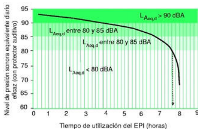
Figura 4 Variación del PNR con el tiempo de utilización del protector auditivo
