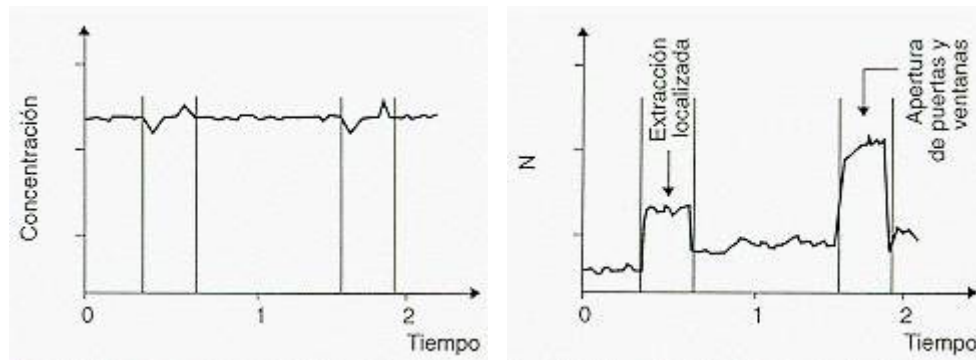
Fig. 3: Método de la concentración constante
