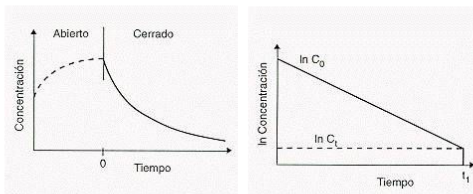
Fig. 1: Método de la caída de la concentración
