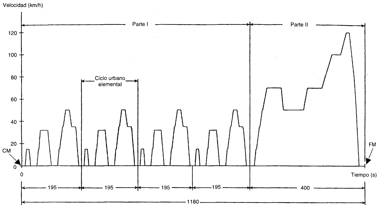
Figura III.1.1 Ciclo de funcionamiento para la prueba de tipo I
