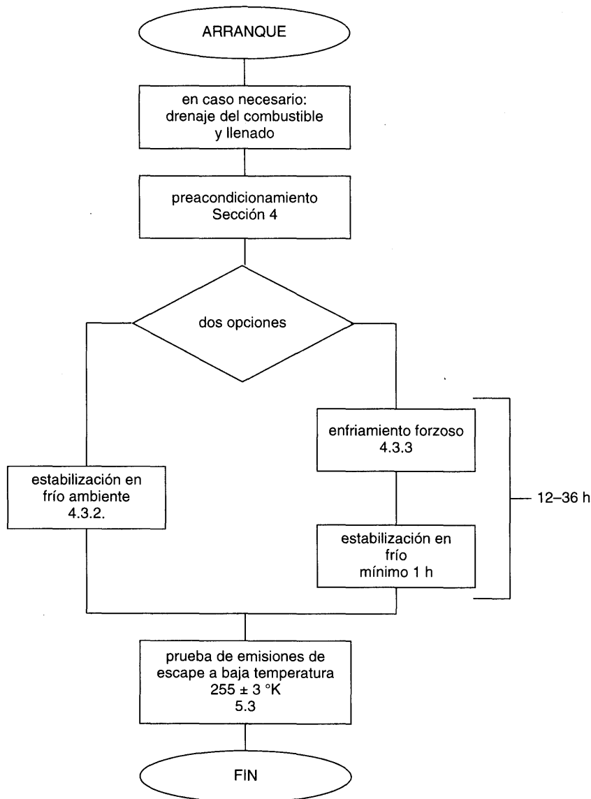
Figura VII.1 Procedimiento para una prueba a baja temperatura ambiente
