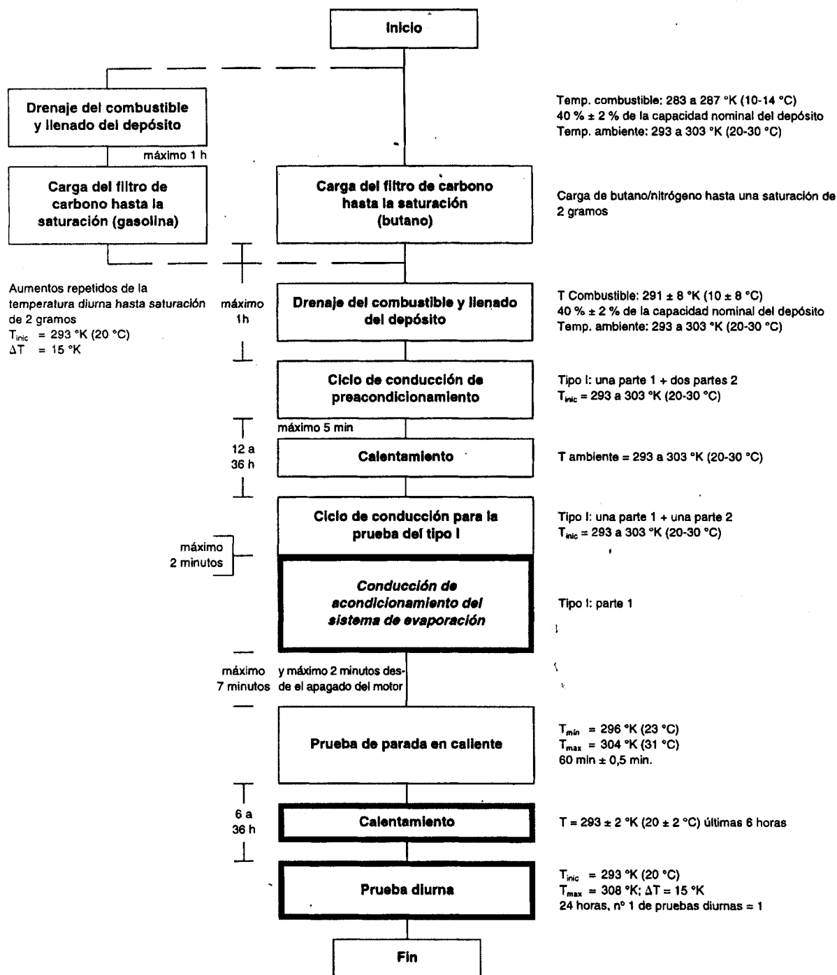
Figura VI.1 Determinación de las emisiones evaporantes Rodaje de 3 000 kilómetros (purgado y carga normales) Control del envejecimiento del filtro(s) de carbono Limpieza al vapor del vehículo (en caso necesario)
