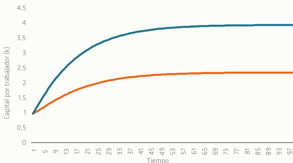
Gráfico 1: Dinámica del capital por trabajador en un modelo teórico de Solow
