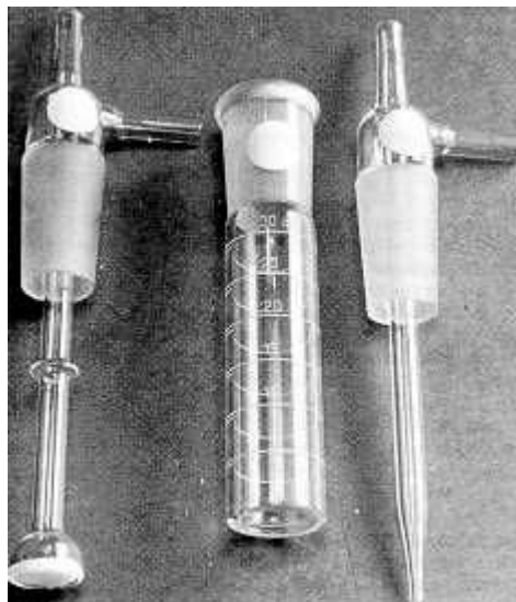
Fig. 1: Componentes impinger
