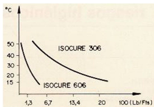
Cambio de viscosidad con la temperatura
