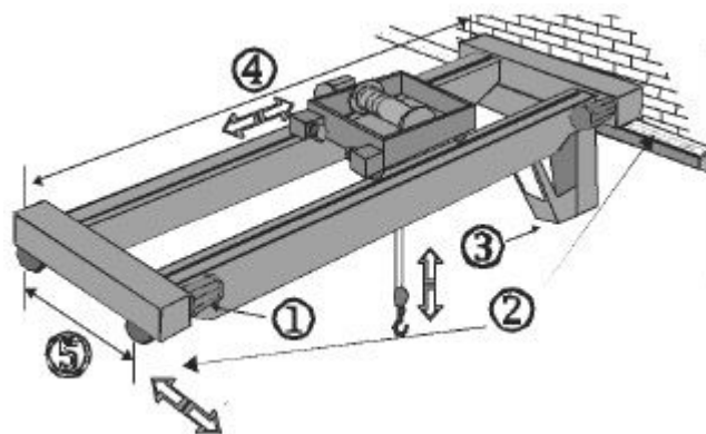
Figura 1 Grúa puente
