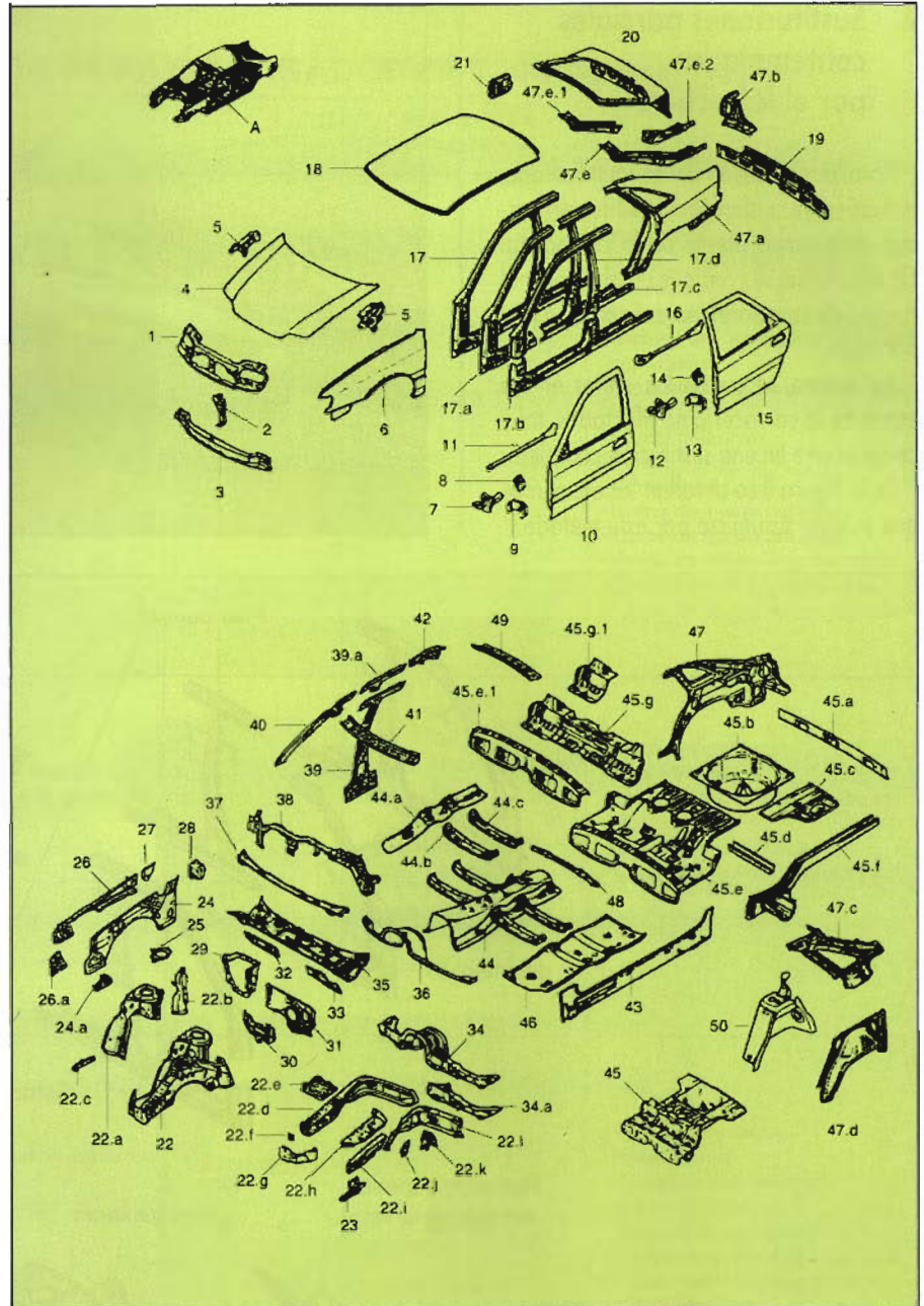
Figura 7. Elementos de la carrocería que suministra el fabricante.
