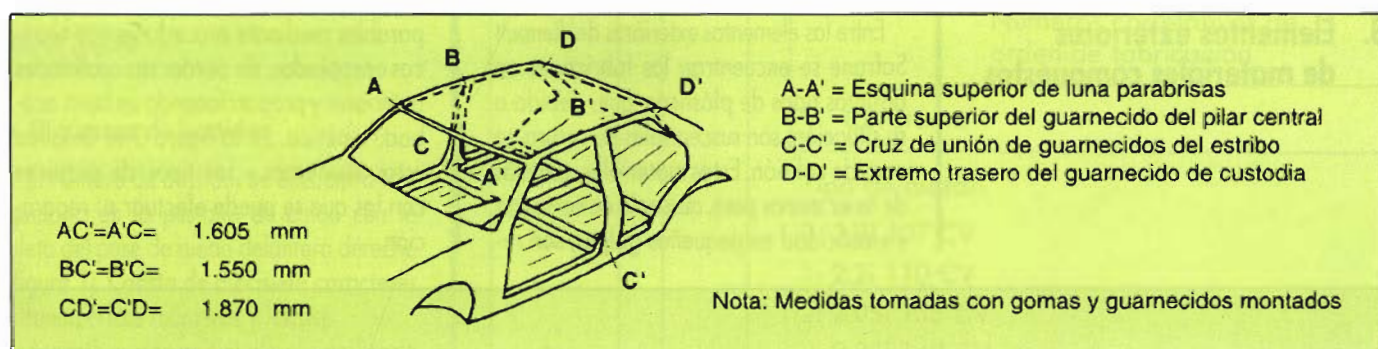
Figura 5. Dimensiones del habitáculo
