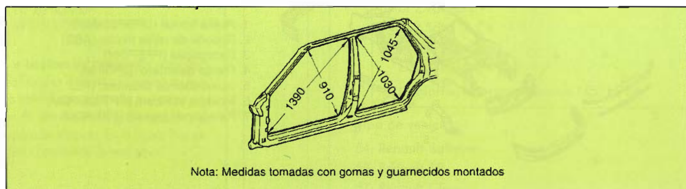
Figura 6. Medidas de los huecos de puertas
