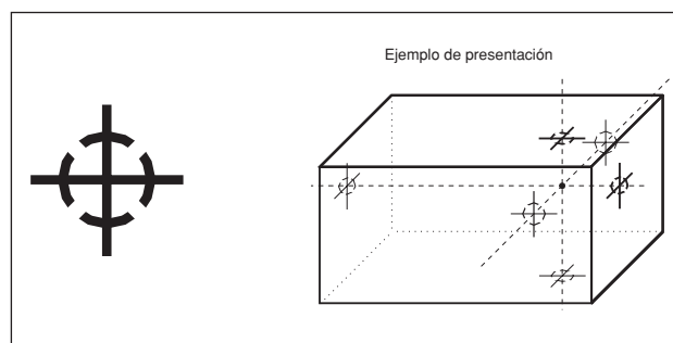
Figura 11 – Señalización del centro de gravedad de una carga.
