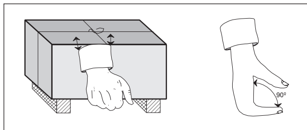
Figura 7 – Agarre regular.
