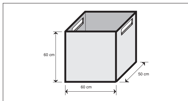
Figura 10 – Tamaño máximo recomendable de una carga.
