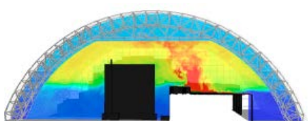
Simulación del incendio (Chernobil)
