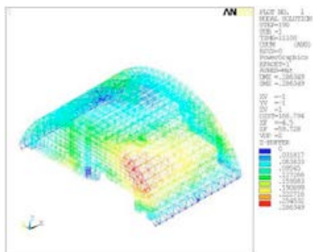
Acciones térmicas sobre la estructura de acero (Chernobil)
