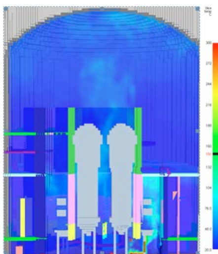
Temperaturas en el edificio del reactor (CIGEO)
