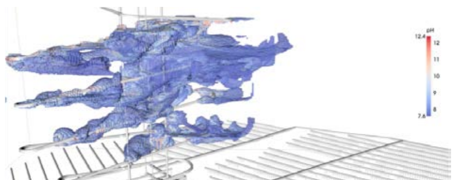
Modelización acoplada hidro-geoquímica para la predicción de la durabilidad del grout de cemento usado para la impermeabilización de las fracturas en el almacenamiento subterráneo de combustible gastado de Forsmark, Suecia. Proyecto realizado para SKB (Suecia).
