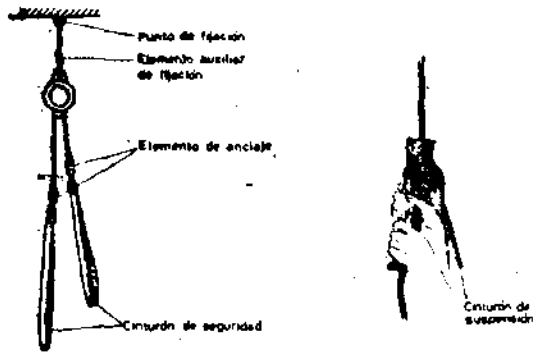
Fig. 3.- EJEMPLOS DE DISPOSITIVOS PARA OPERACIONES DE DESCENSO. EVACUADORES O DESCENDEDORES
