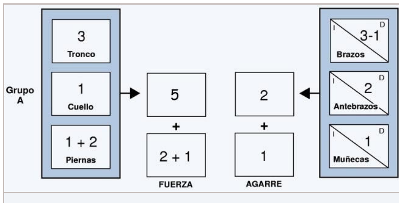
FIGURA 8 Ejemplo práctico: Hoja de puntuación. Adaptado de Hignett, S., McAtamney, L. (2000) Applied Ergonomics , 31, 201-5.
