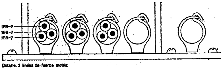
Detalle. 3 líneas de fuerza motriz
