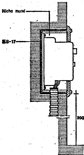
Sección
