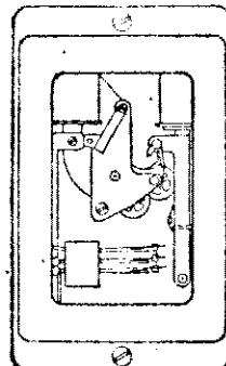
Alzado
