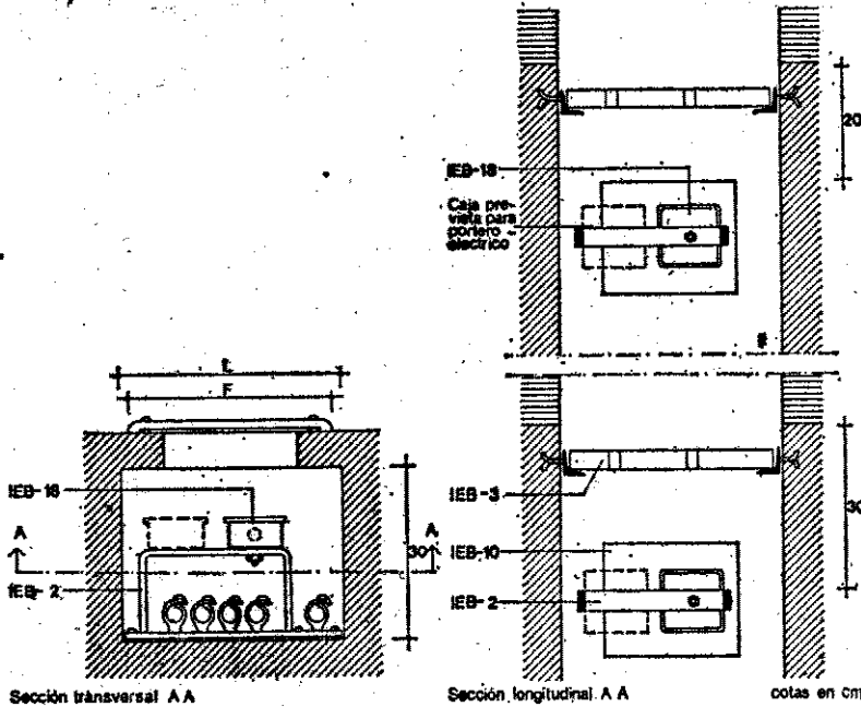
Sección transversal A A
