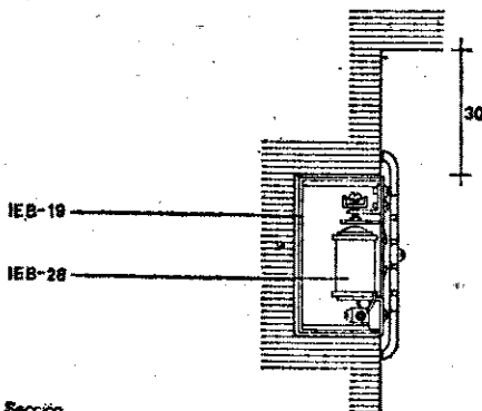
Sección
