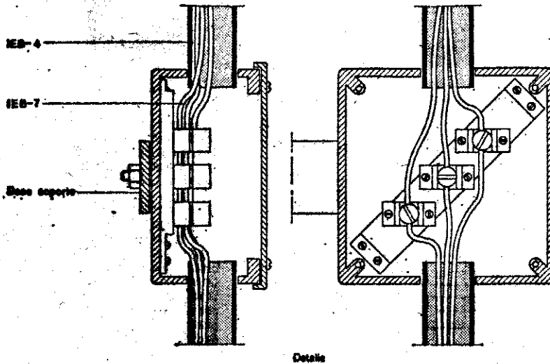
Detalle
