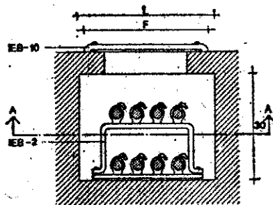
Sección transversal
