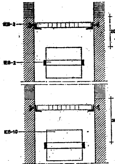
Sección longitudinal A-A
