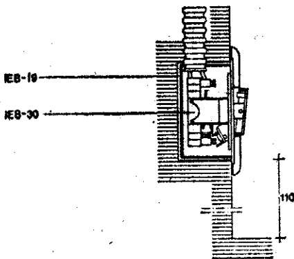
Sección
